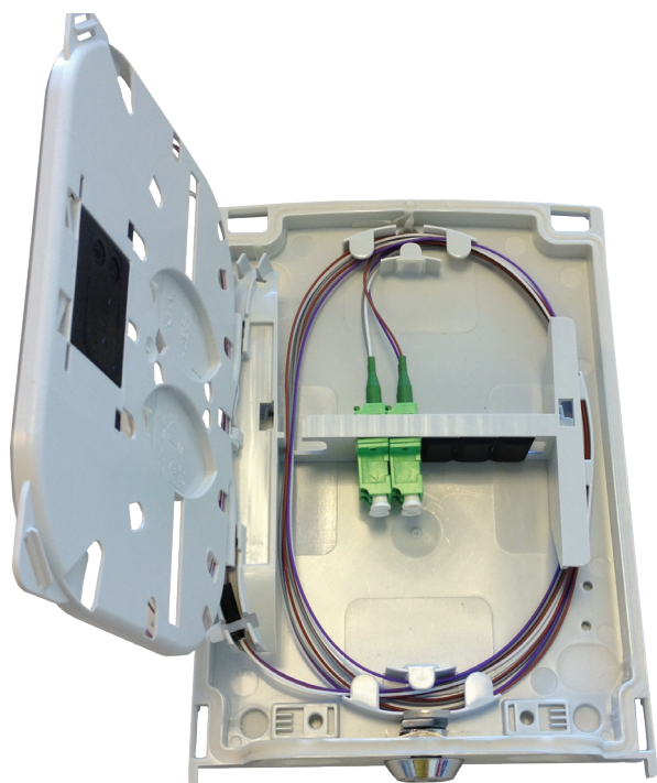
FTTx Wandverteiler OTB12 spleißfertig bestückt mit 4 x LC/APC
