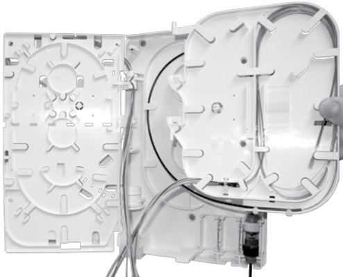
LWL APL mit herausgenommener Spleisskassette
