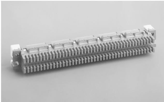
LSA-PLUS-Erddrahtleiste, 84-polig
